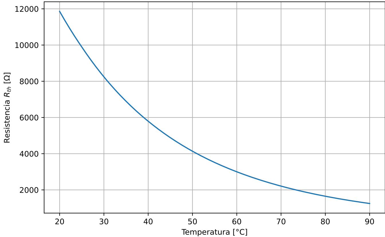
Resistencia del termistor vs Temperatura
